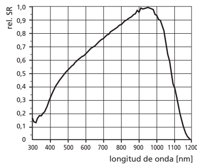
Curva característica de la sensibilidad espectral.
